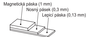
Obr.3 Pořadí montáže
