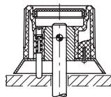
Montáž pomocí příčného kolíku a odpruženého trnu s nastavitelným tlakem
