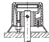
Montáž pomocí příčného kolíku a odpruženého šroubu s pojistnou maticí
