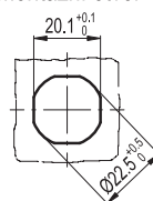
Montážní otvor
