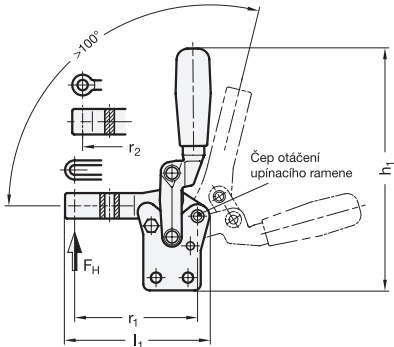
Princip ovládání
