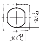
Montážní otvor
