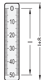
Posloupnost čísel O
