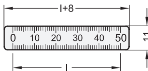
Posloupnost čísel L
