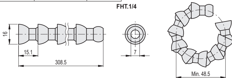
FHT.1/4
