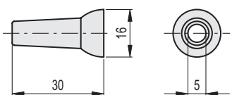
FHN.1/4-B-5
