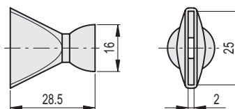
FHN.1/4-P25
