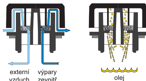
Schéma proudění
